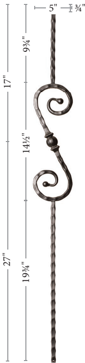
9034HF- * -44 5 pcs per box 225 pcs per skid
