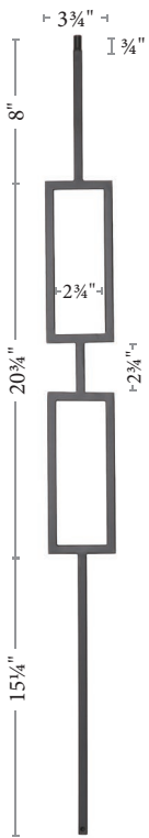
9091CS 5 pcs per box 385 pcs per skid
