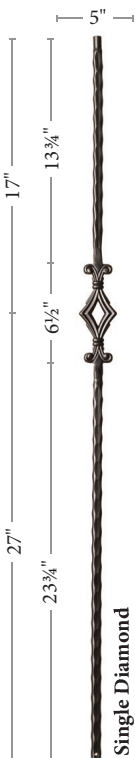
9040HF- * -44 10 pcs per box 420 pcs per skid
