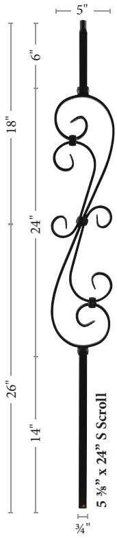
9981TB-SB 5 pcs per box 210 pcs per skid
