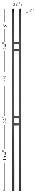
9087CS 10 pcs per box 770 pcs per skid
